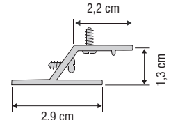
Seitenführung 2,2 / 2,9 cm
