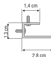
Seitenführung 1,4 / 2,8 cm
